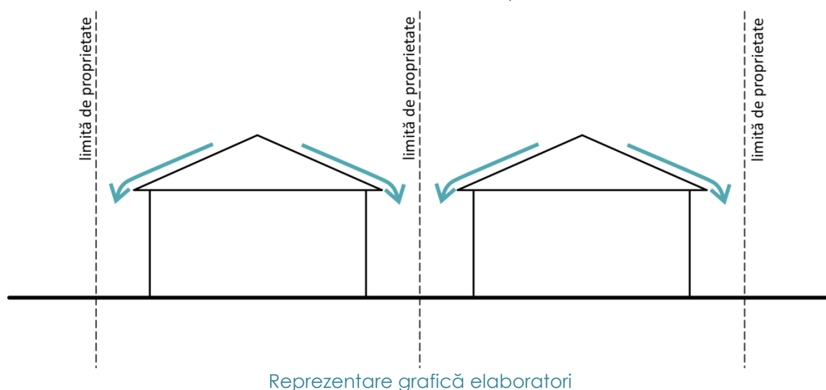
Figura 2 – Picătura streșinii
